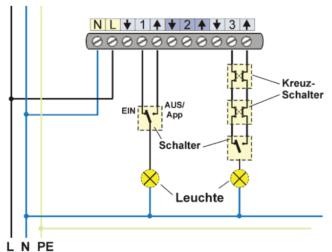
Abbildung 3a: Anschluss Leuchten und Bedienschalter (Ausschnitt)
