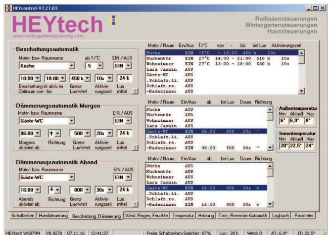
Maske Beschattung, Dämmung: Einrichtung der Beschattungsautomatik sowie der Dämmungsautomatik für Morgen und Abend
