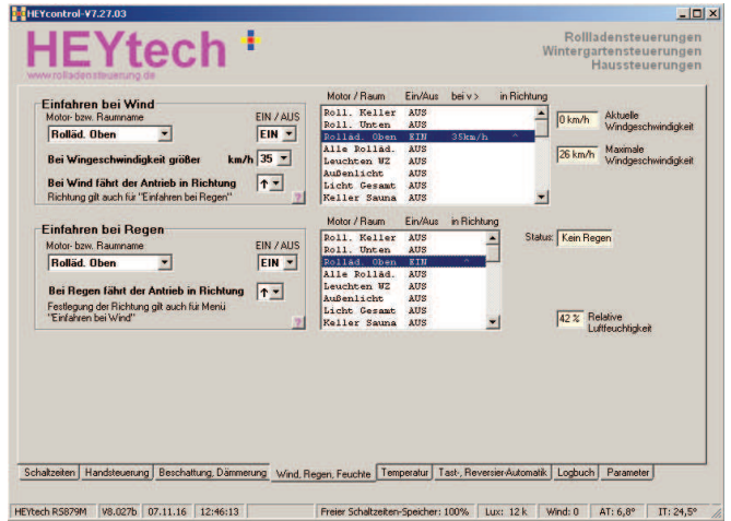
Maske Wind, Regen: Einrichtung der Windsteuerung und der Regensteuerung
