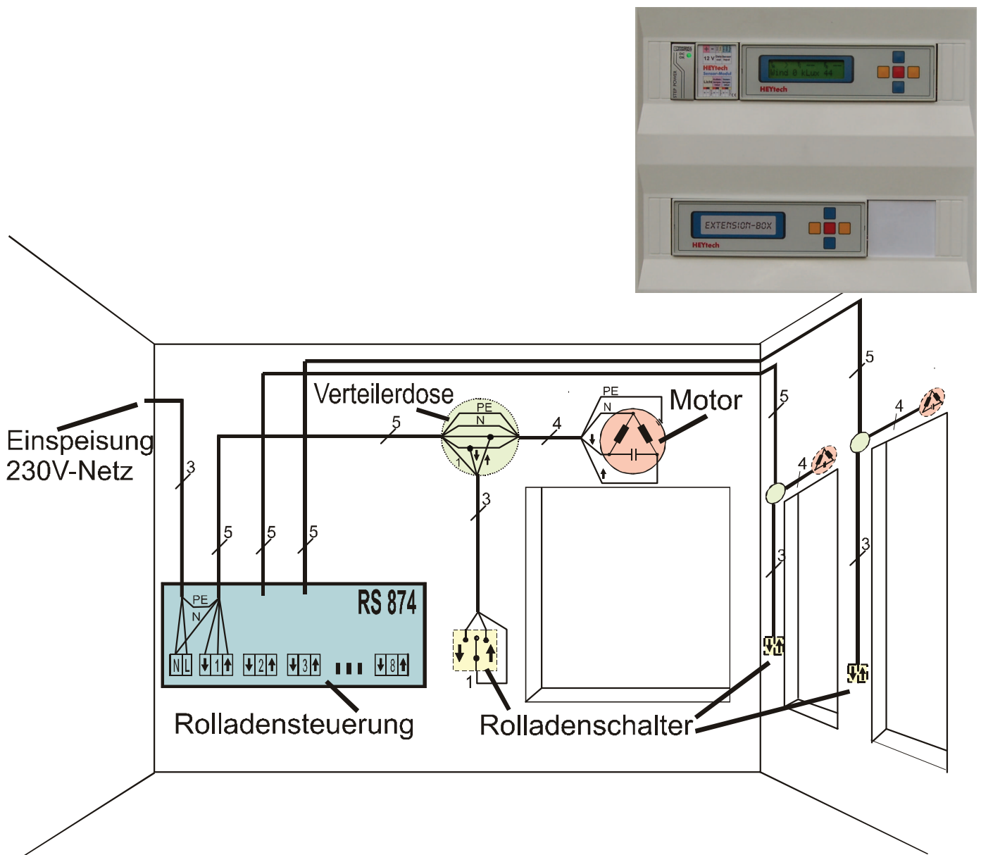
Abbildung 9: Leitungsführung
