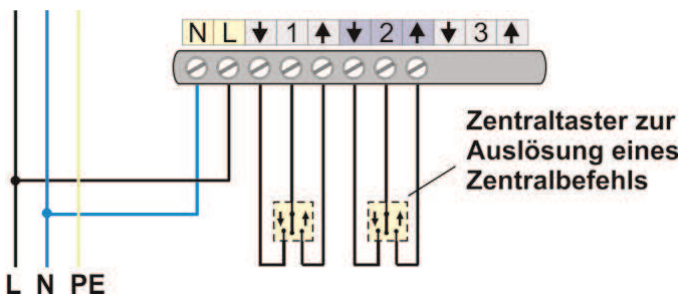
Abbildung 10: Gruppen-Zentraltaster
